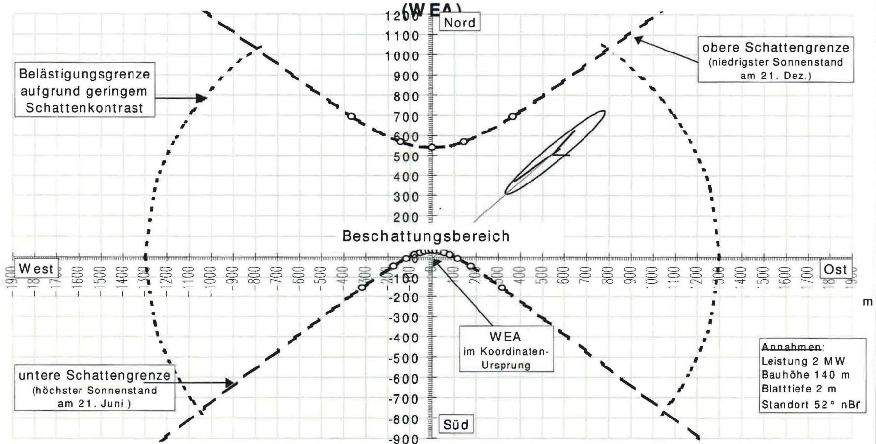
Abb.: Möglicher Beschattungsbereich einer großen Windenergieanlage
